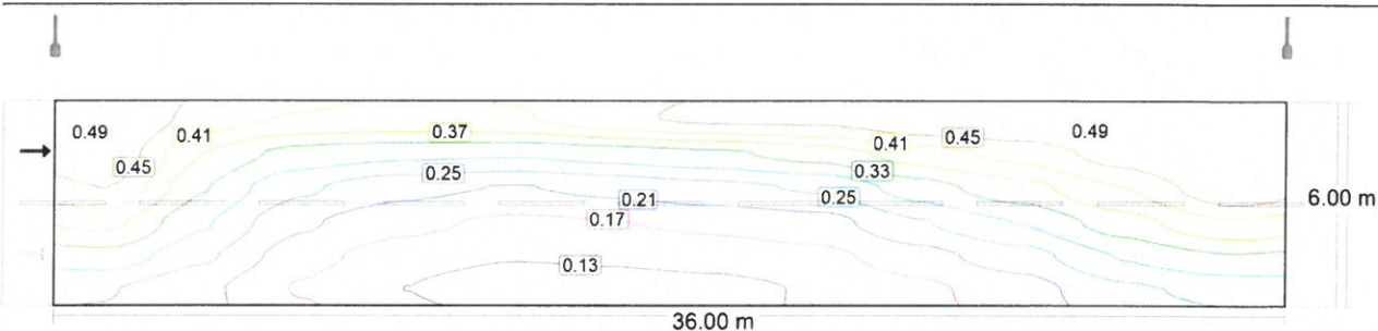
Observator 2: Valoarea de întreținere, densitatea luminii cu carosabil uscat [cd/m²] (Linii Isolux)
