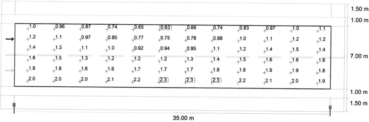
Observator 2: Densitatea luminii la instalația nouă [cd/m²] (Linii Isolux)
